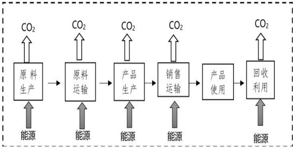
图 2 曲轴产品生命周期评价边界图
